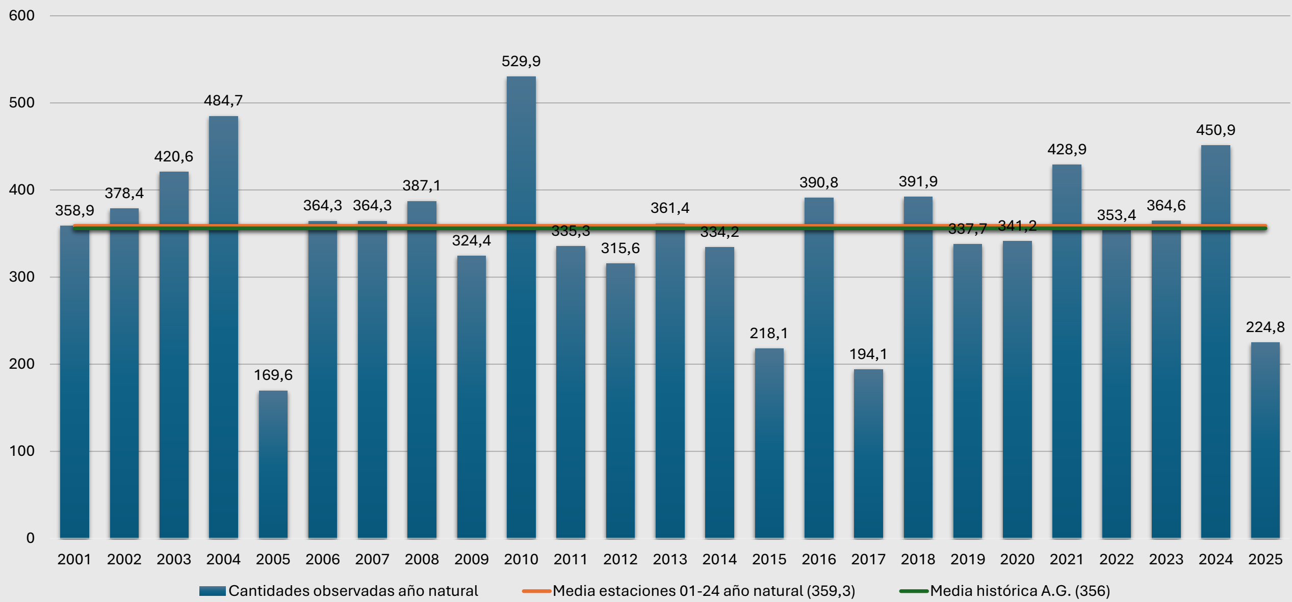
Evolución pluviométrica media AÑO NATURAL (enero-diciembre)
